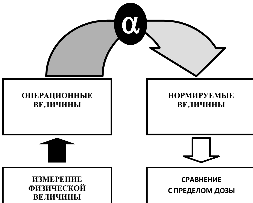
Рис.7.2. Связь между различными величинами, используемыми в радиационной безопасности.
